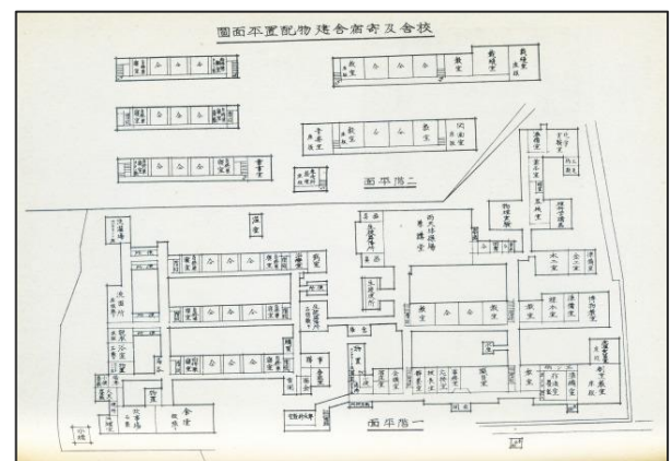
図10 校舎及寄宿舎建物配置平面図
